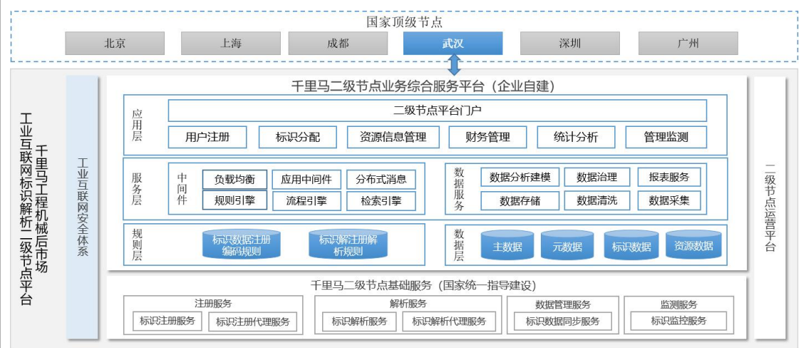
图 5-3 千里马工业互联网标识解析二级节点平台示意图
