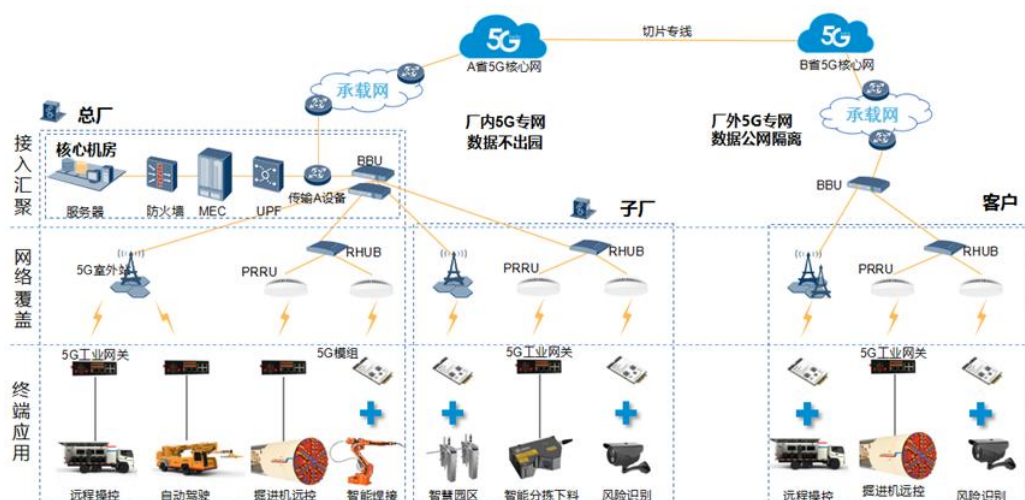
图 4-6 网络方案示意图
