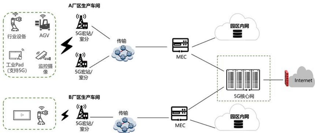
图 4-5 跨园区 5G 专网部署
