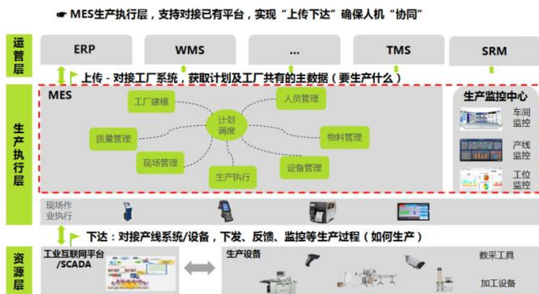
图 6-4 中联重科 MES 平台部署实施图
