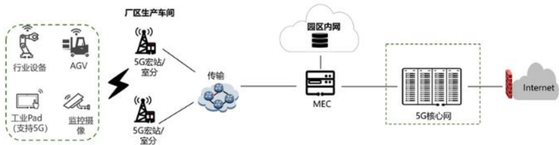
图 4-4 园区 5G 专网部署
