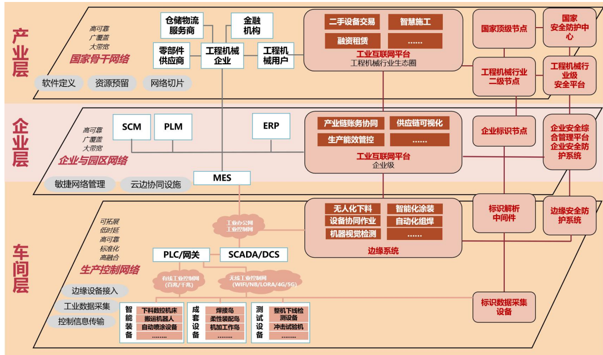
图 3-2 工程机械行业工业互联网融合创新实施架构 8
